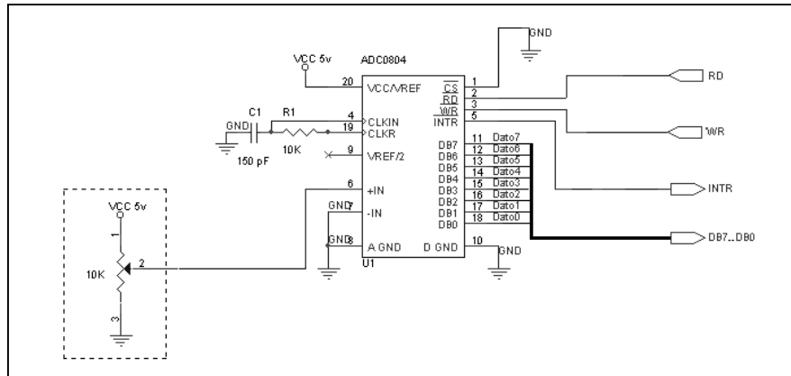
Figura 4. Diagrama del convertidor conectado al puerto paralelo.
