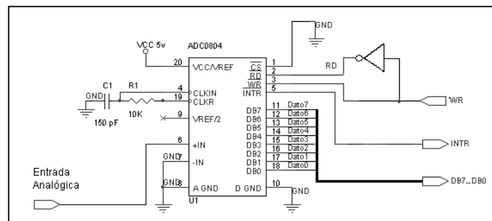
Figura 8. Conexión Free Running para el ADC0804.
